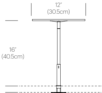
CIRCA GROMMET
